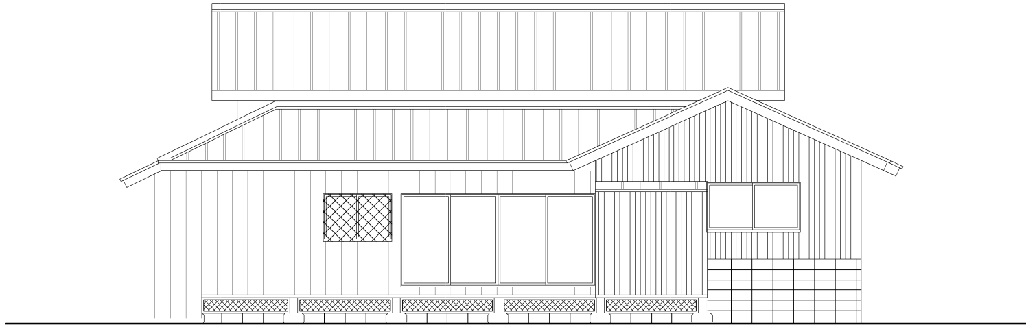
北側立面図
