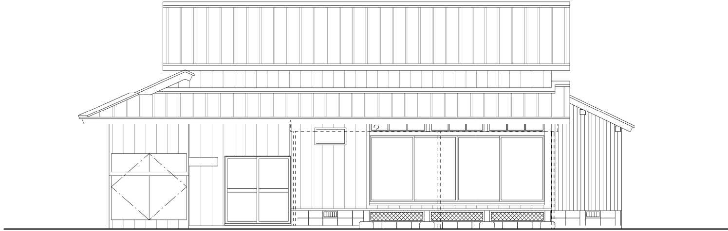
南側立面図
