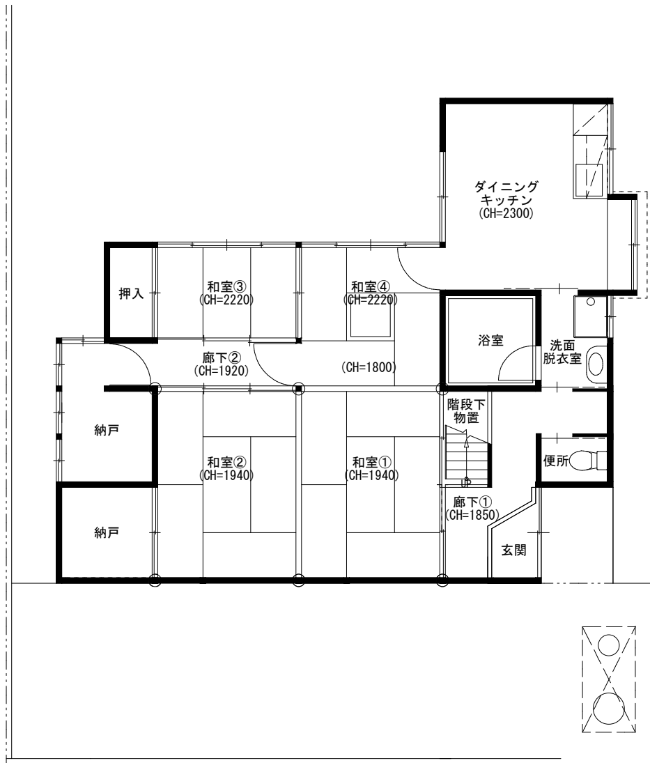
【平面図】
