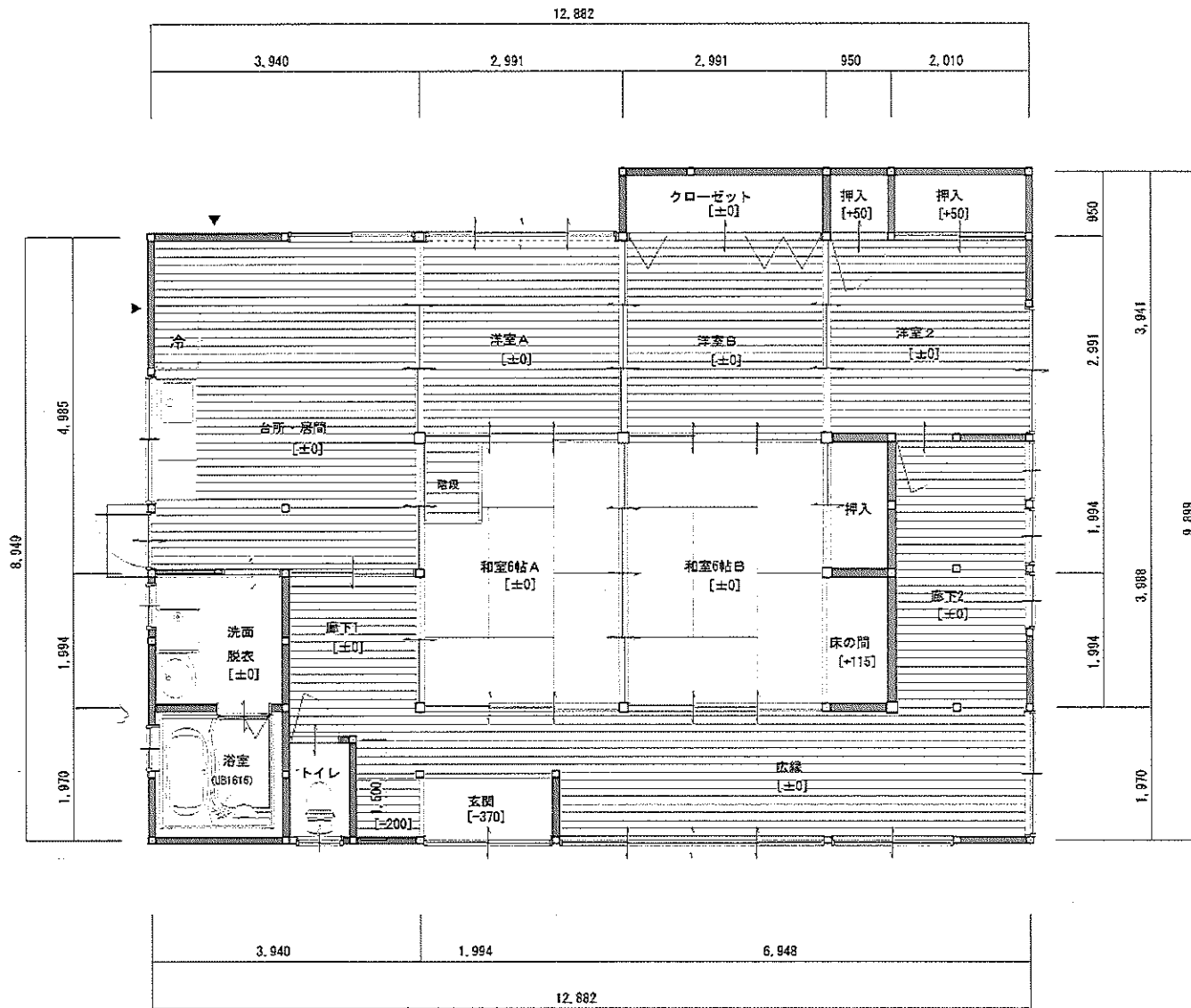
平面図
